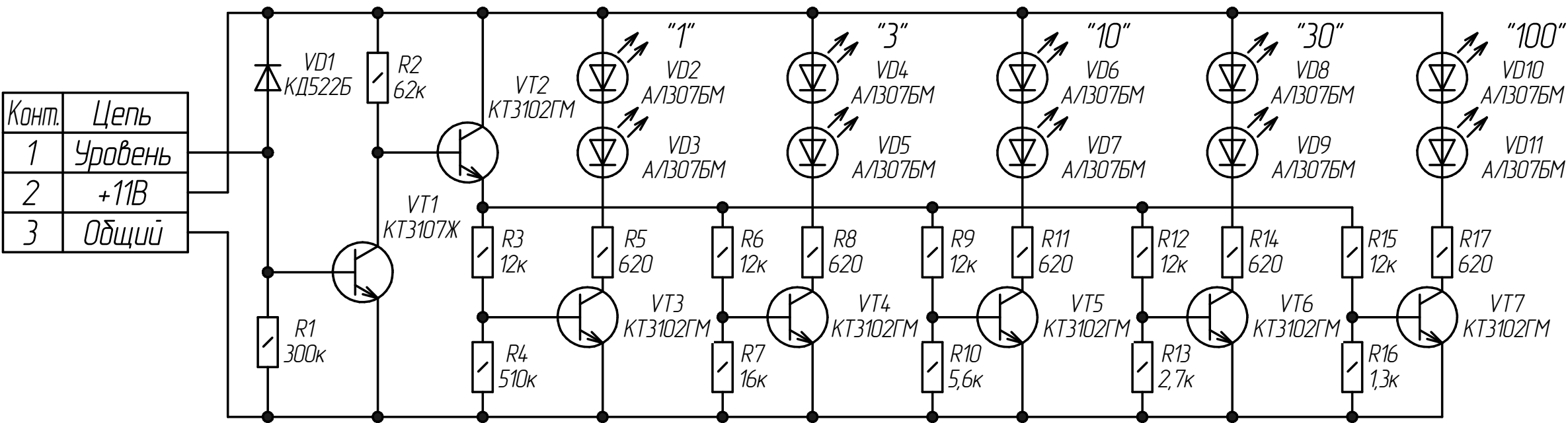
Индикатор уровня ИУ
