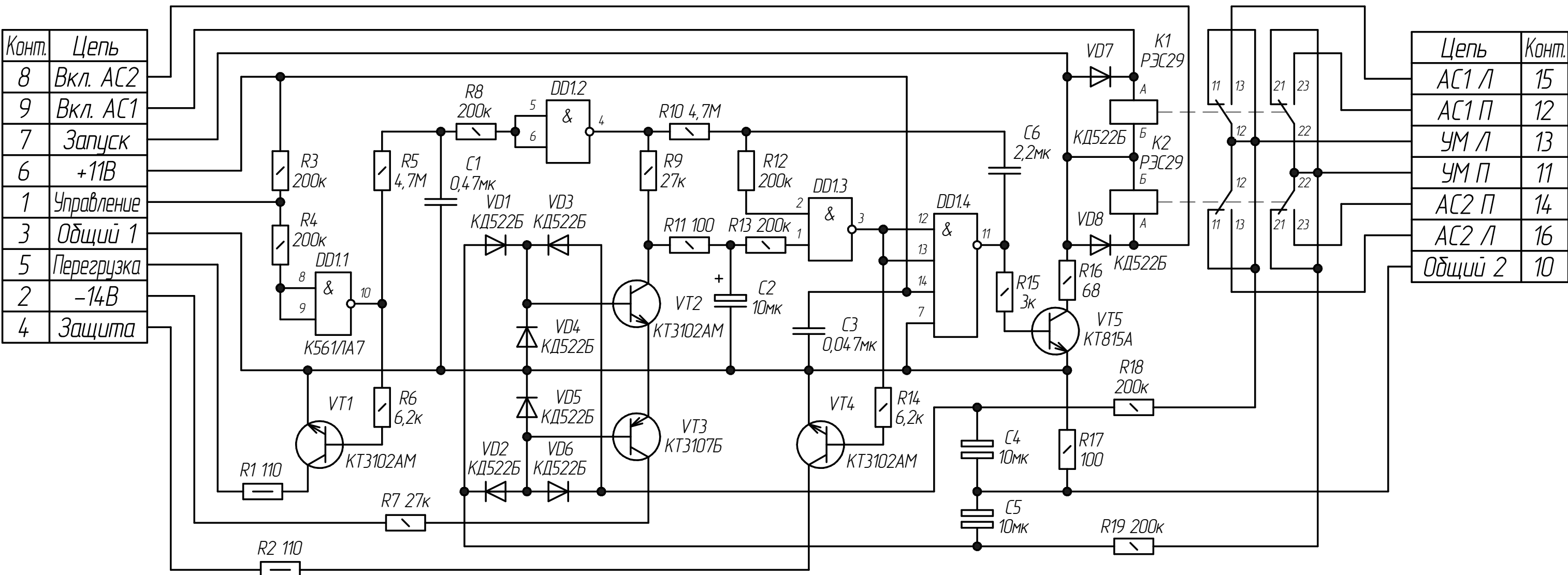
Комплексная защита КЗ
